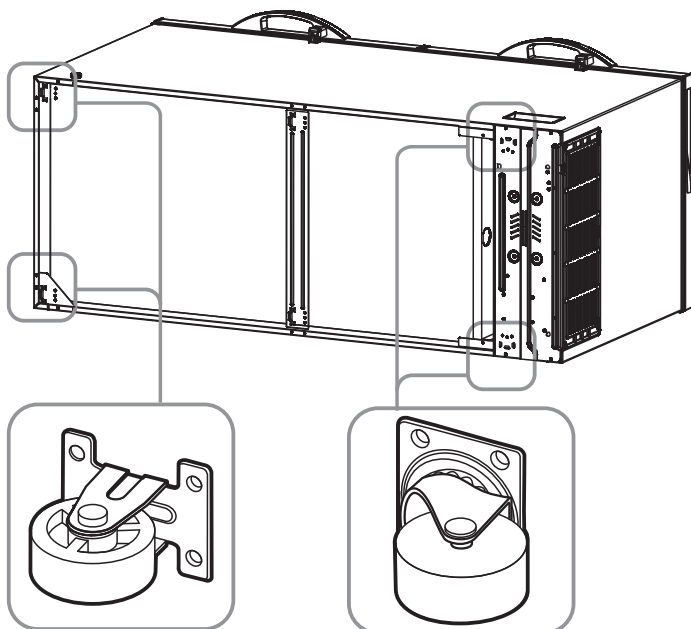
Ruedas direccionales
