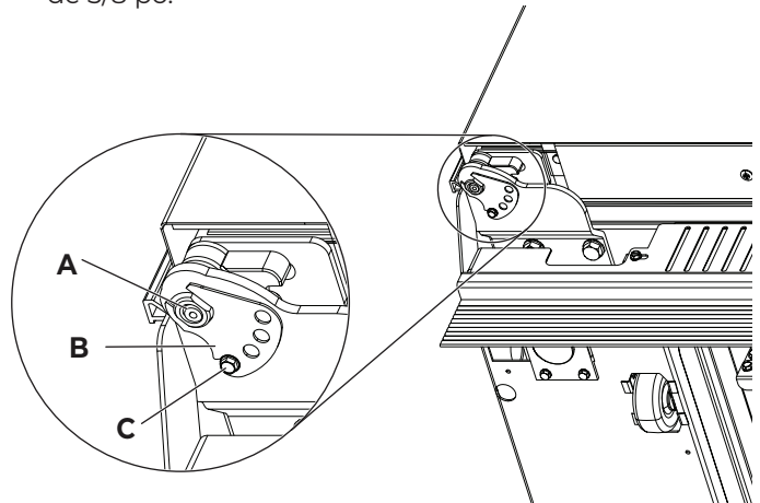
A. Bague B. Plaque de verrouillage C. Vis de butée de porte
