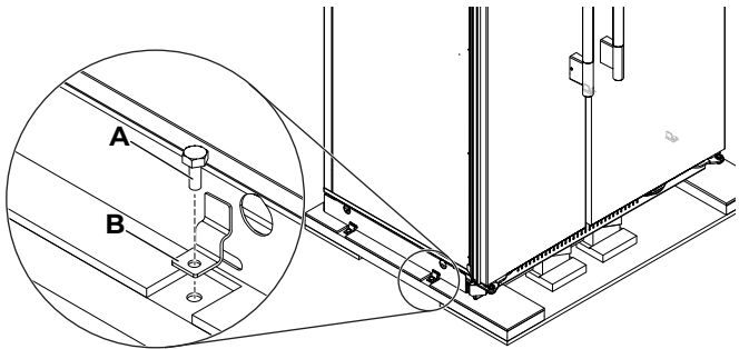
A. Screws B. Brackets
