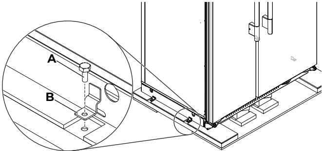
A. Tire-fonds B. Supports
