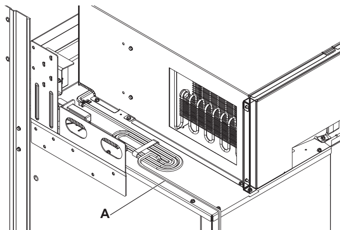
A. Cordon d'alimentation
