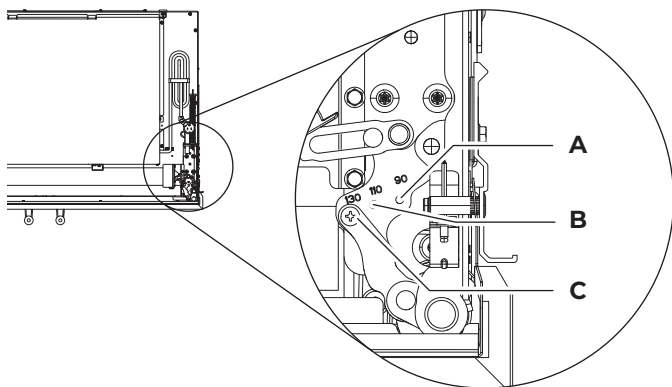
A. Position 90° B. Position 110° C. Position 130° vis de réglage de l'ouverture de la porte
