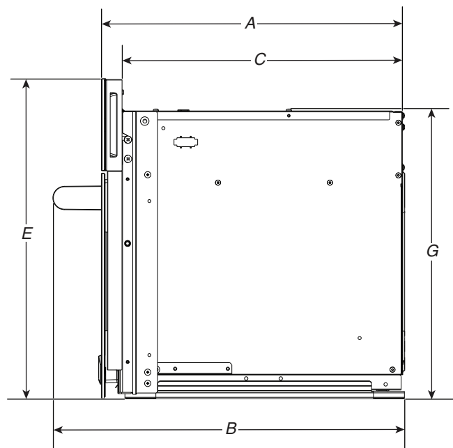
VISTA LATERAL
