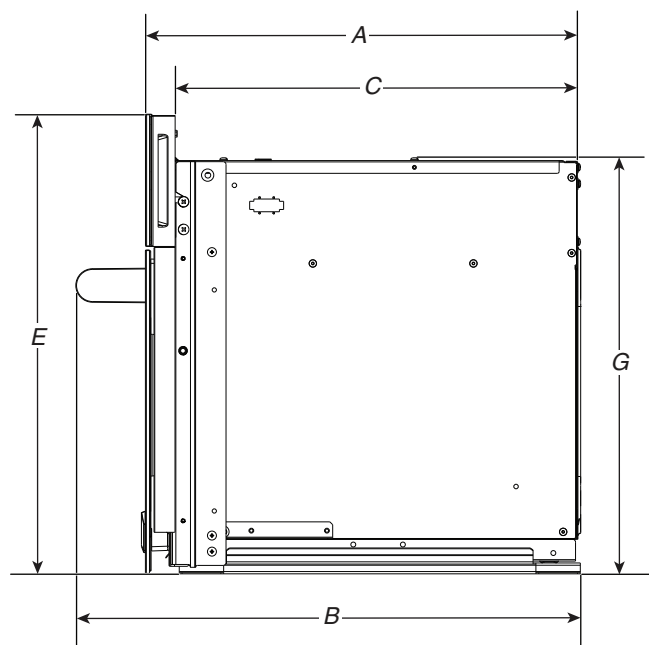
VUE LATÉRALE
