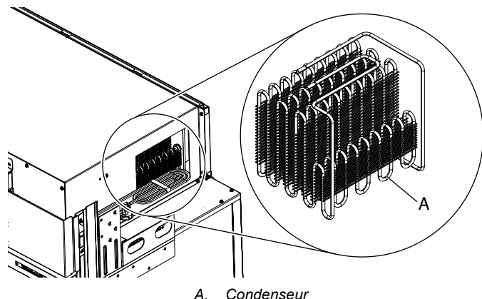
A. Condenseur
