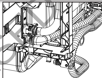
Ubicación de la manguera de desagüe
