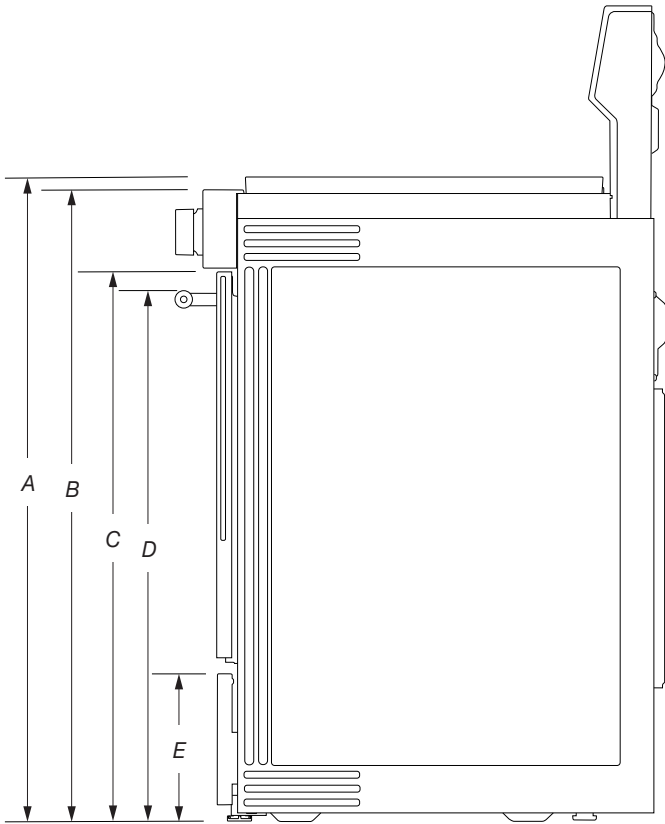
VISTA LATERAL
