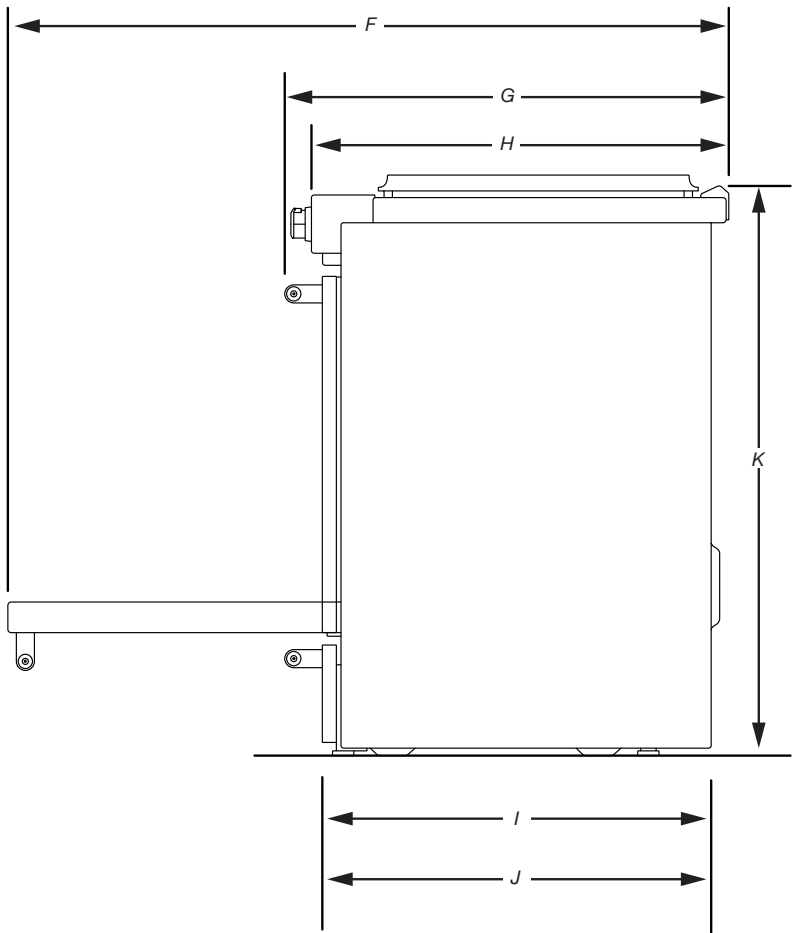
VUE LATÉRALE
