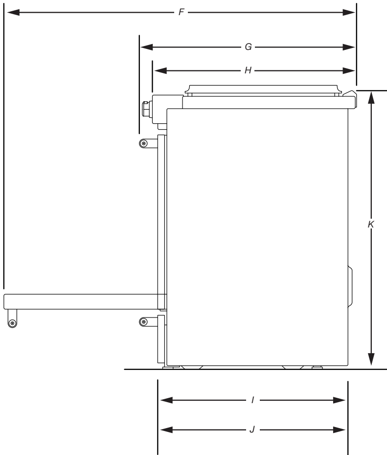
VISTA LATERAL
