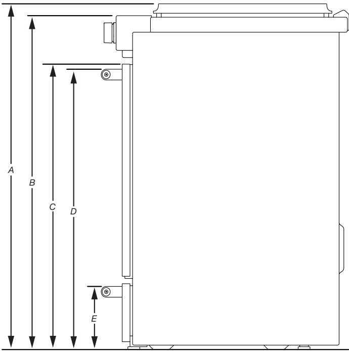
VISTA LATERAL
