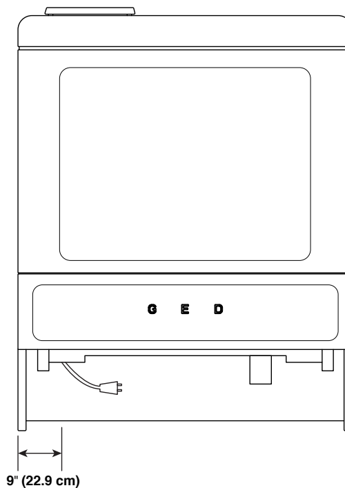
VUE ARRIÈRE
