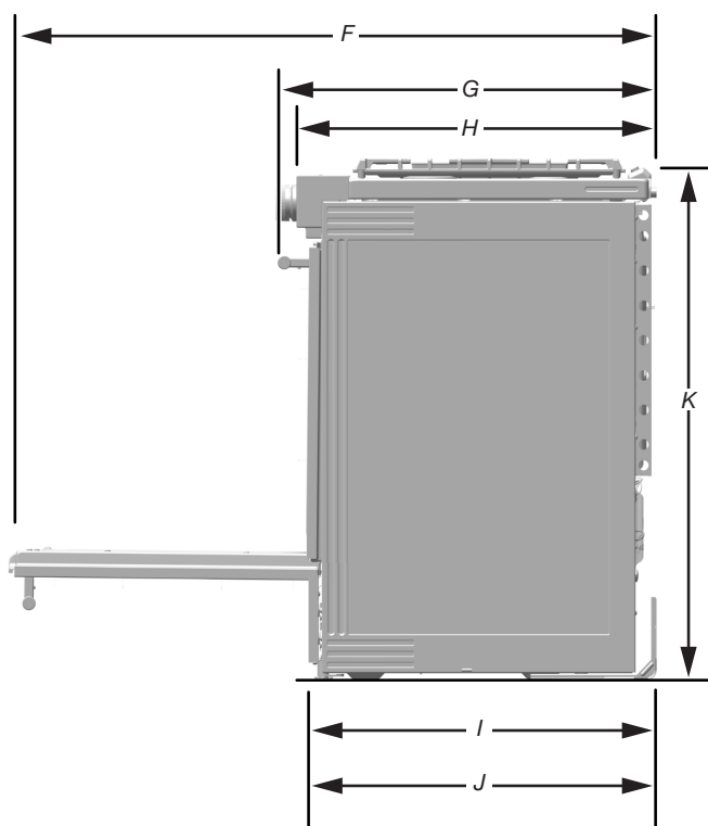
VUE LATÉRALE
