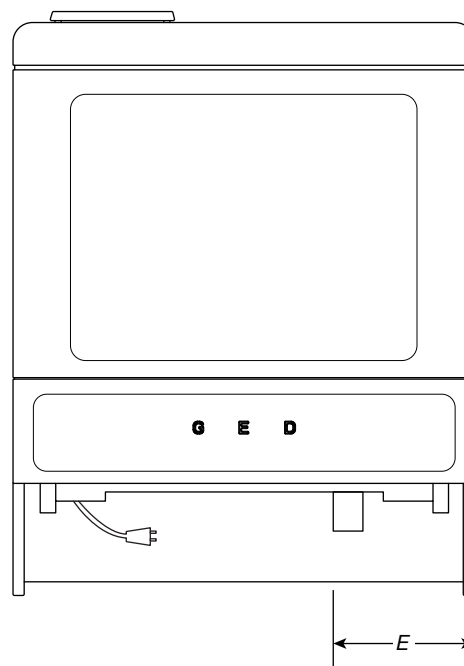
VUE ARRIÈRE
