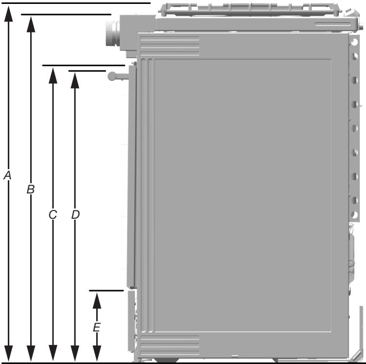
VISTA LATERAL
