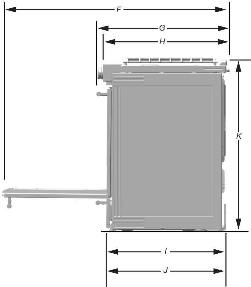
VISTA LATERAL
