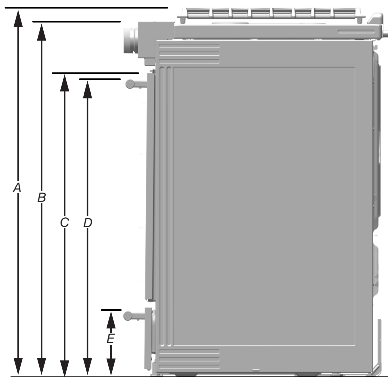
VUE LATÉRALE
