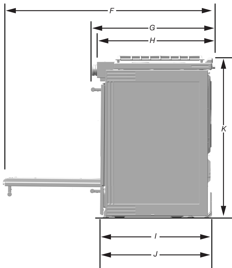
VUE LATÉRALE
