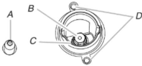
A. Électrode d'allumage B. Injecteur C. Porte-injecteur D. Vis
