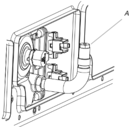
A. Injecteur
