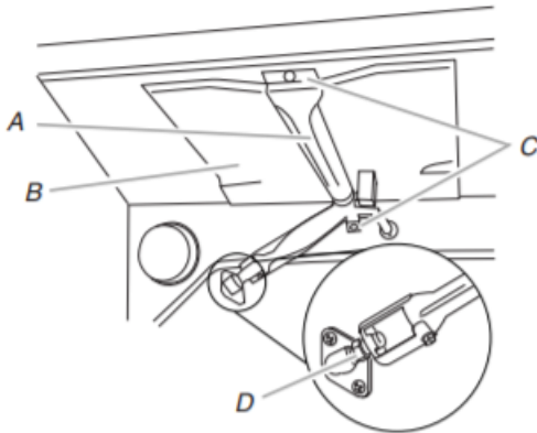
A. Brûleur du grill B. Répartiteur de flammes C. Vis D. Injecteur
