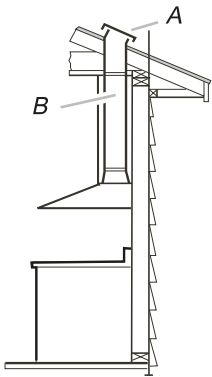
A. Bouche de décharge sur toit B. Conduit dia. 6 po (15,2 cm)
