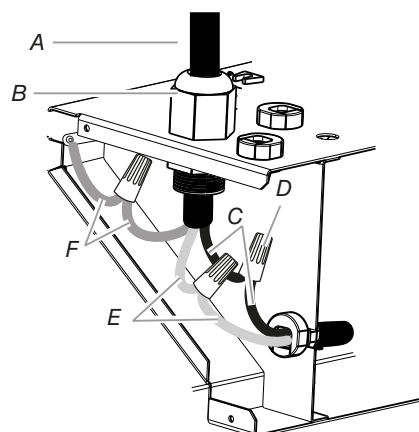
A. Cable alimentación de la casa B. Alivio de tensión aprobado por UL o CSA. C. Cables negros D. Conectores aprobados por UL E. Cables blancos F. Cables verdes o amarillo/verdes
