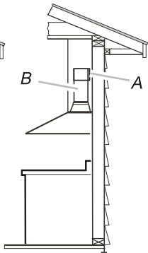
A. Déflecteur B. Conduit dia. 6 po (15,2 cm)
