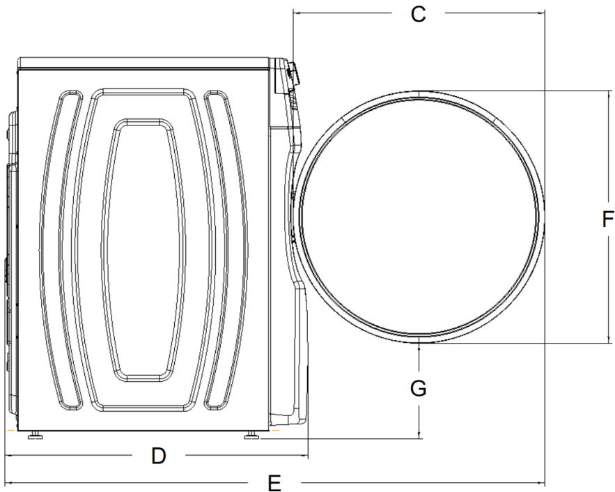
VUE LATÉRALE
