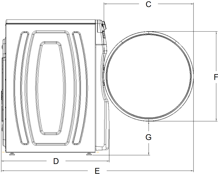
VISTA LATERAL
