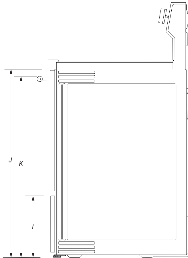
VUE LATÉRALE
