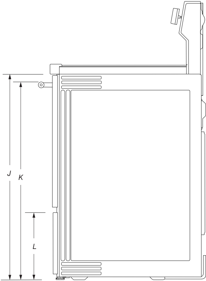
VISTA LATERAL
