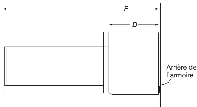
VUE LATÉRALE 1
